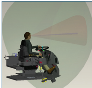
Vision Cones
